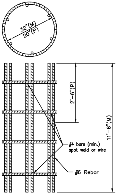
REBAR CAGE
