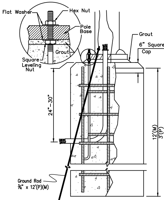
REBAR CAGE
